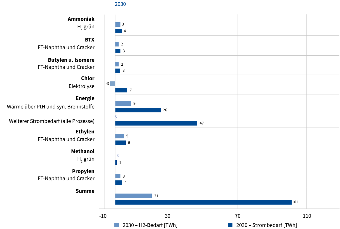
Abbildung 17: Wasserstoff- und Strombedarf nach Szenario 3
