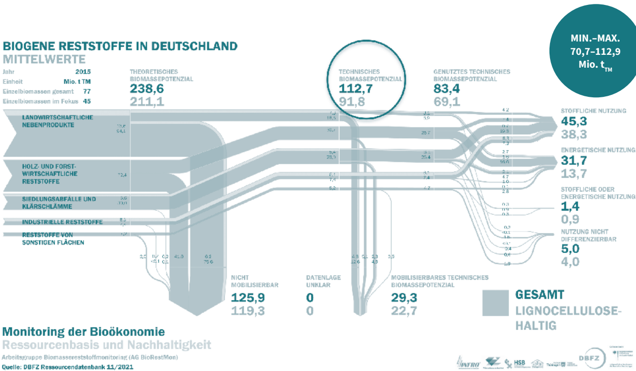
Abbildung 6: Stoffstrom von 77 biogenen Rest- und Abfallstoffen (inklusive des jeweiligen Anteils der lignocellulosehaltigen Rest- und Abfallstoffe) 2015 in Deutschland 24
