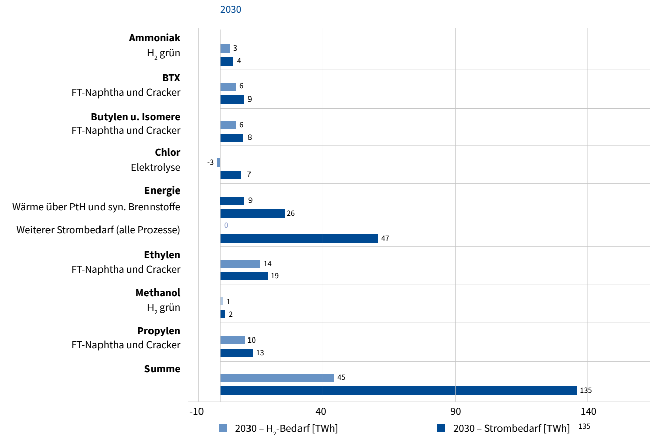
Abbildung 14: Wasserstoff- und Strombedarf nach Szenario 2
