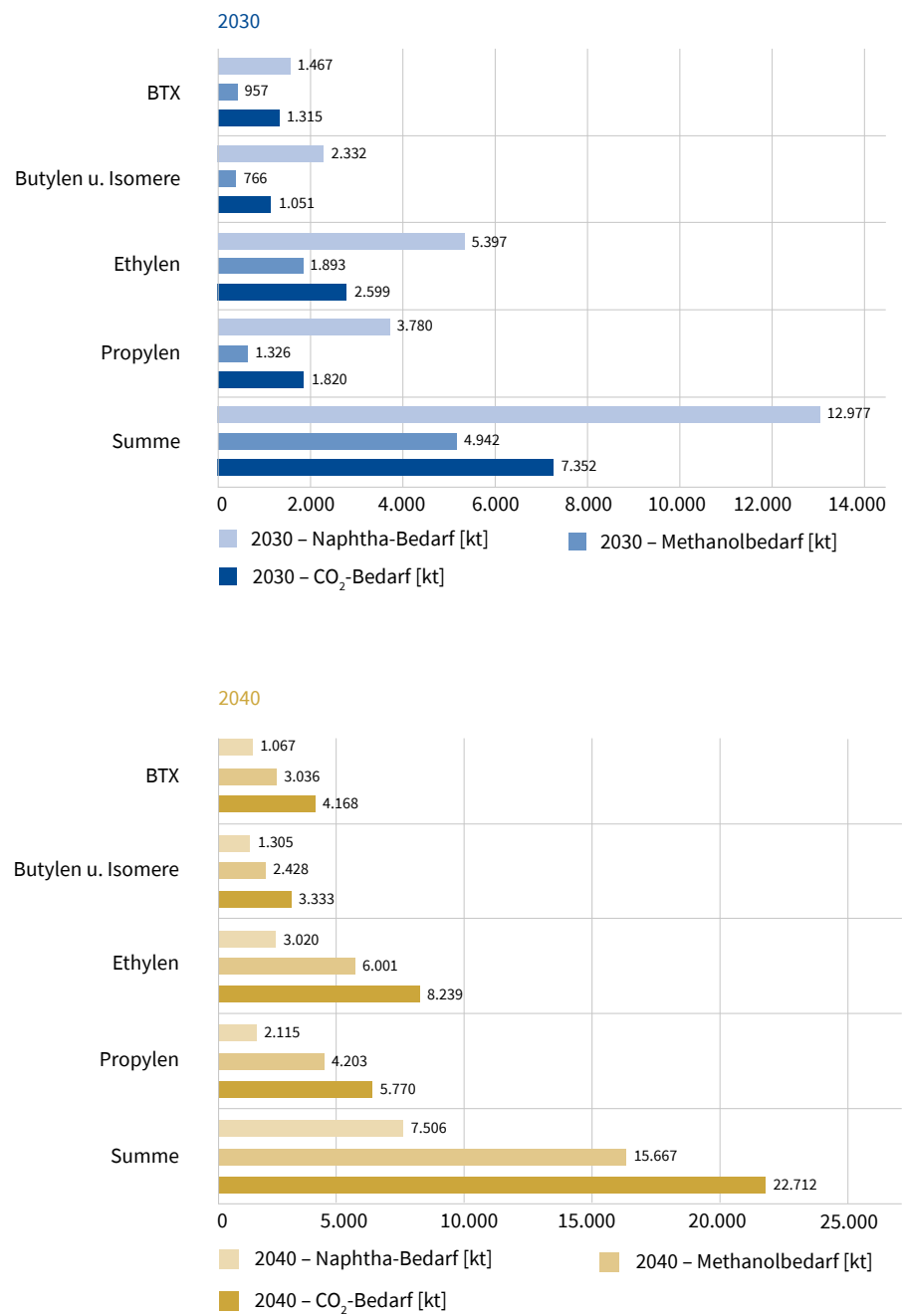
Abbildung 12: Rohstoffbedarf für Olefine und Aromaten nach Szenario 1
