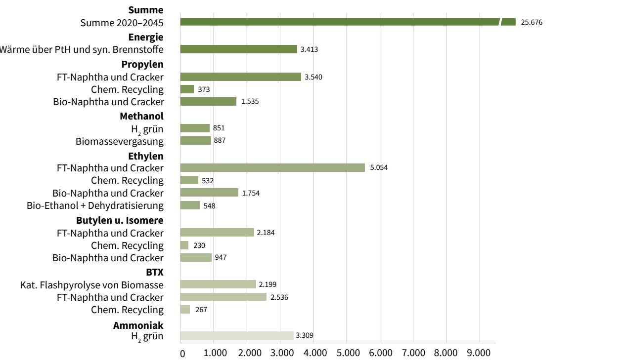
Abbildung 19: Nominaler Investitionsbedarf bis 2045 in Mio. € für Szenario 3
