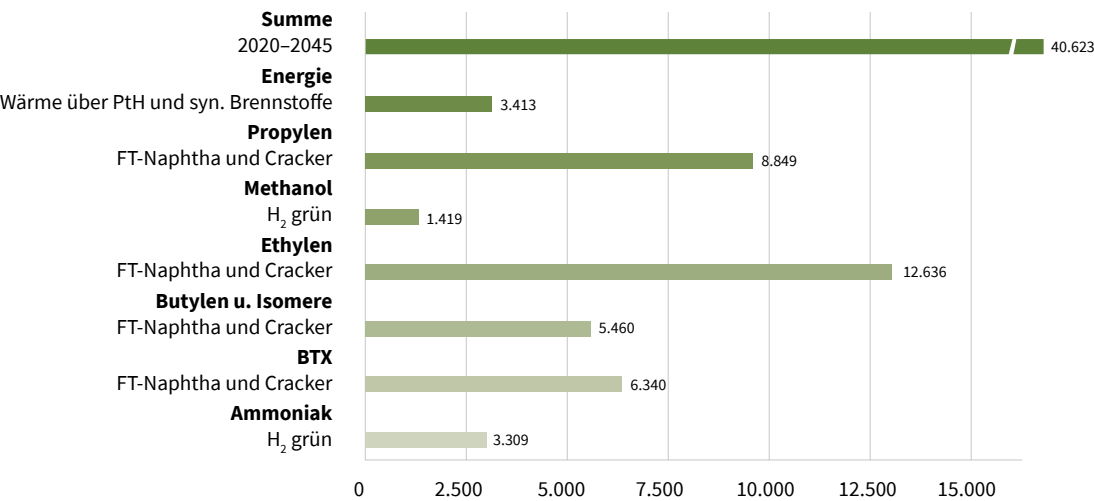
Abbildung 16: Nominaler Investitionsbedarf bis 2045 für Szenario 2
