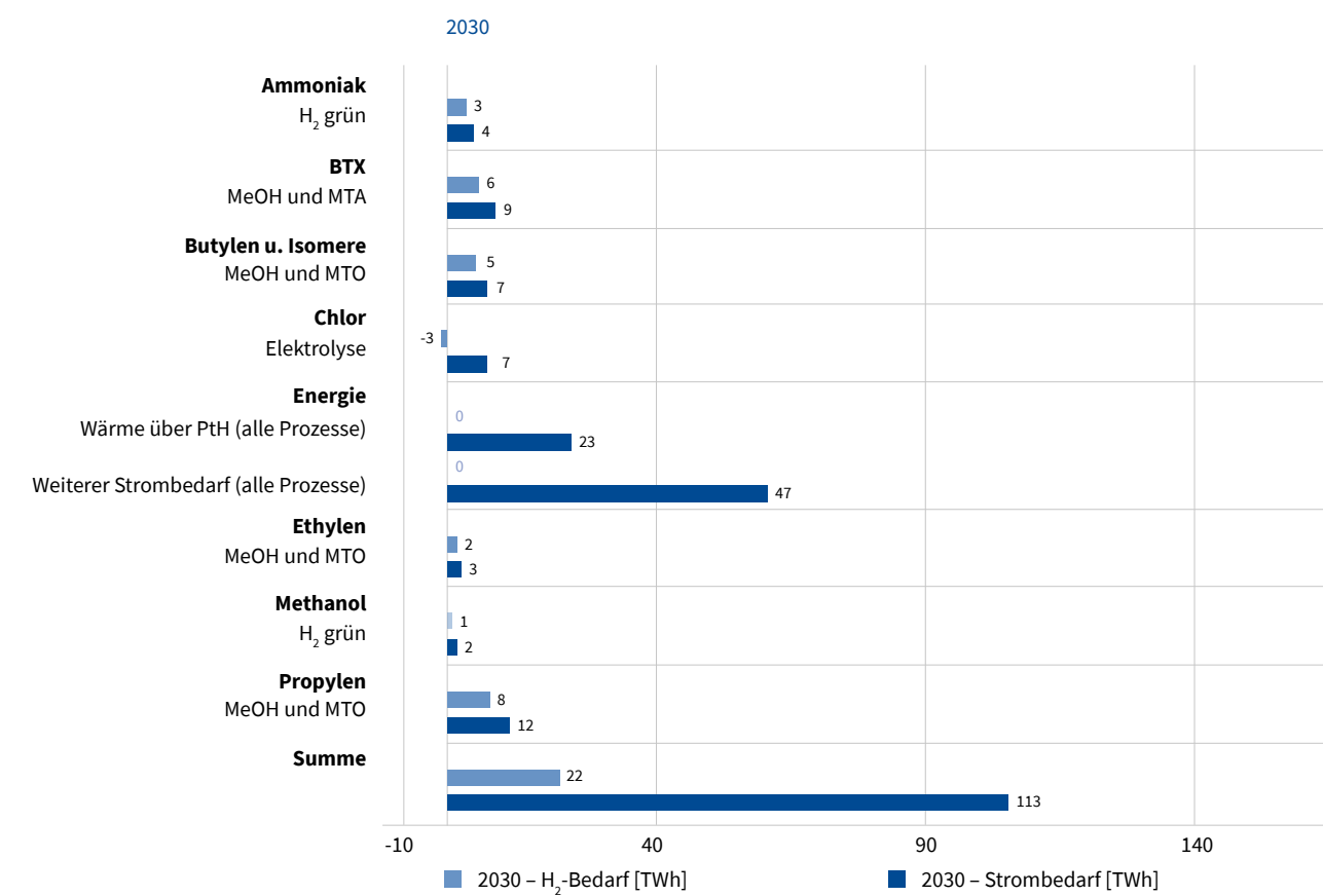
Abbildung 11: Wasserstoff- und Strombedarf nach Szenario 1
